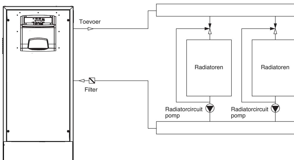
Ketelcircuit met meerdere groepen radiatoren.
