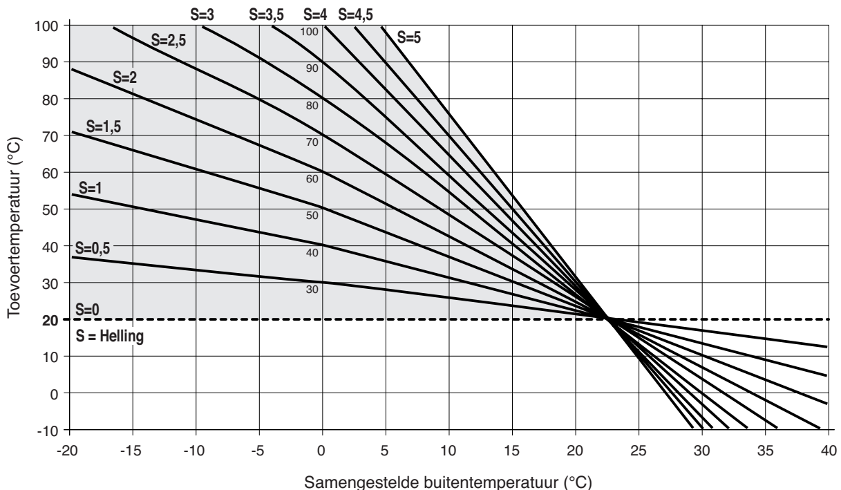
Stookcurven met setpoint omgevingstemperatuur = 20°C
