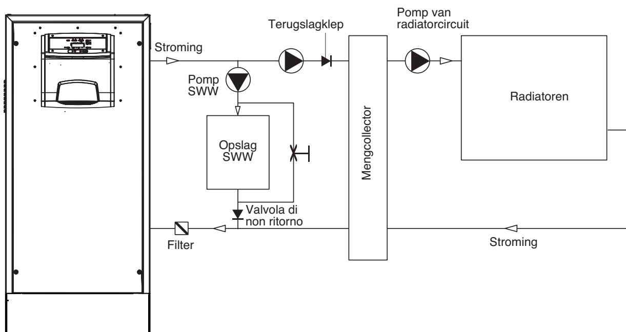
Ketelcircuit met pomp SWW (productie ketel > productie SWW) en 1 groep radiatoren
