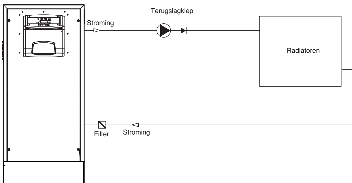
Ketelcircuit met een groep radiatoren
